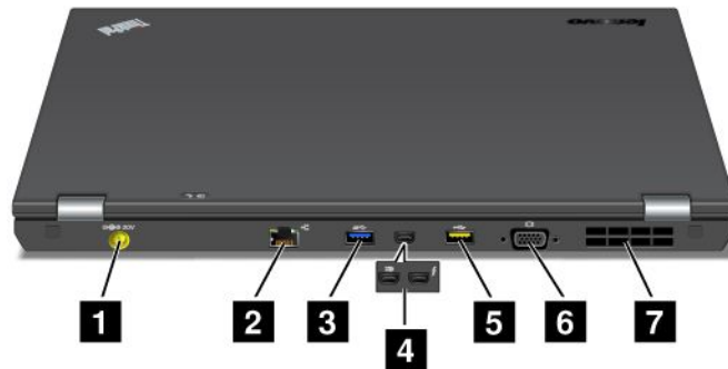
Abbildung 5. Rückansicht des ThinkPad T430s und T430si
