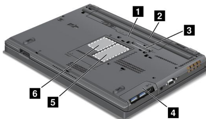
Abbildung 4. Ansicht des ThinkPad T430 und T430i von unten
