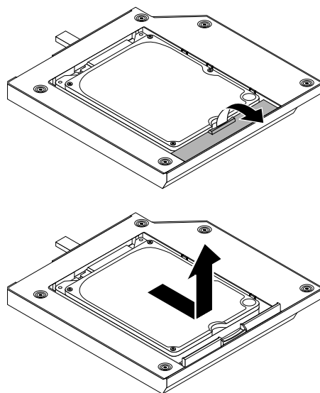
Abbildung 28. Das sekundäre Festplattenlaufwerk vom Adapter entfernen
