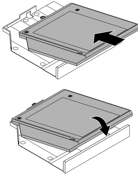
Abbildung 31. Adapter für das Festplattenlaufwerk in der Adapterhalterung installieren
