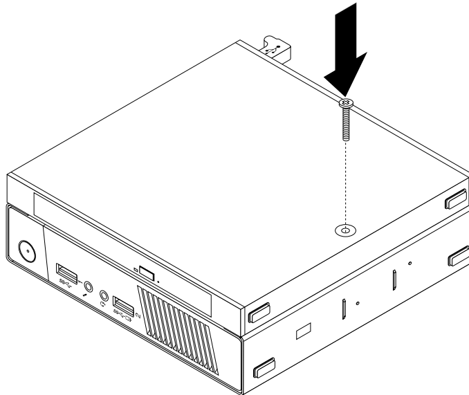
Abbildung 24. Schraube anbringen, mit der das Gehäuse für das optische Laufwerk gesichert ist
