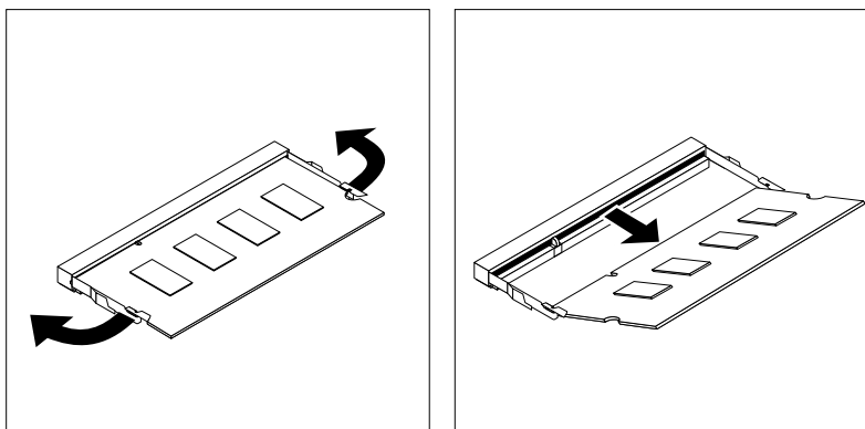
Abbildung 43. Speichermodule entfernen
