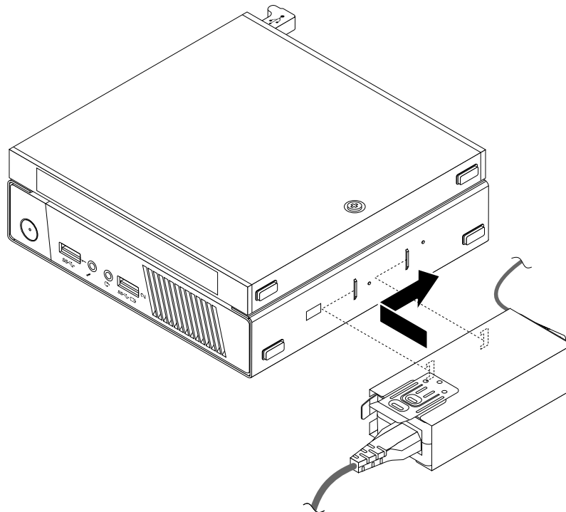
Abbildung 16. Netzteilhalterung installieren
