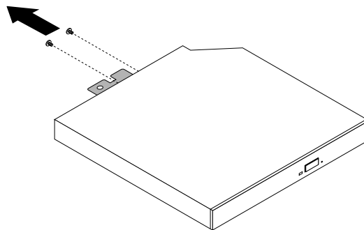
Abbildung 19. Metallplatte des optischen Laufwerks entfernen
