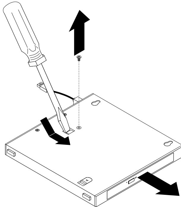
Abbildung 18. Optisches Laufwerk aus dem Gehäuse für das optische Laufwerk entfernen
