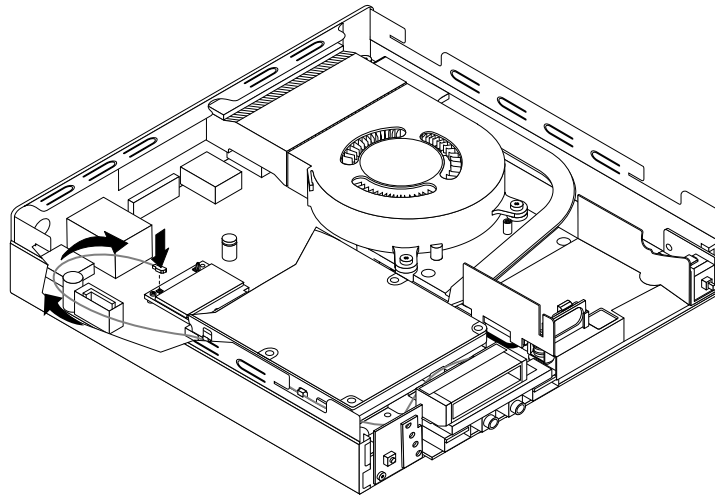
Abbildung 56. Kabel der vorderen Wi-Fi-Antenne anbringen
