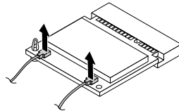
Abbildung 49. Kabel des Wi-Fi-Kartenmoduls entfernen
