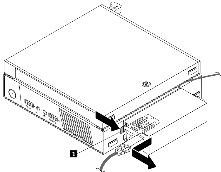
Abbildung 15. Netzteilhalterung entfernen
