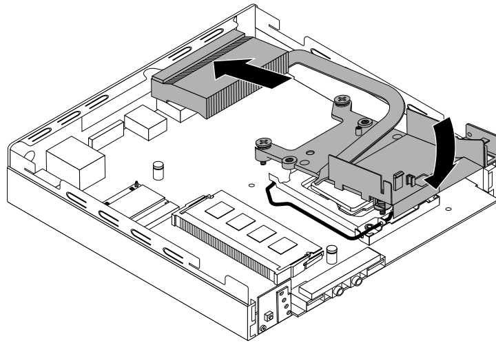
Abbildung 69. Neues Temperaturmodul positionieren
