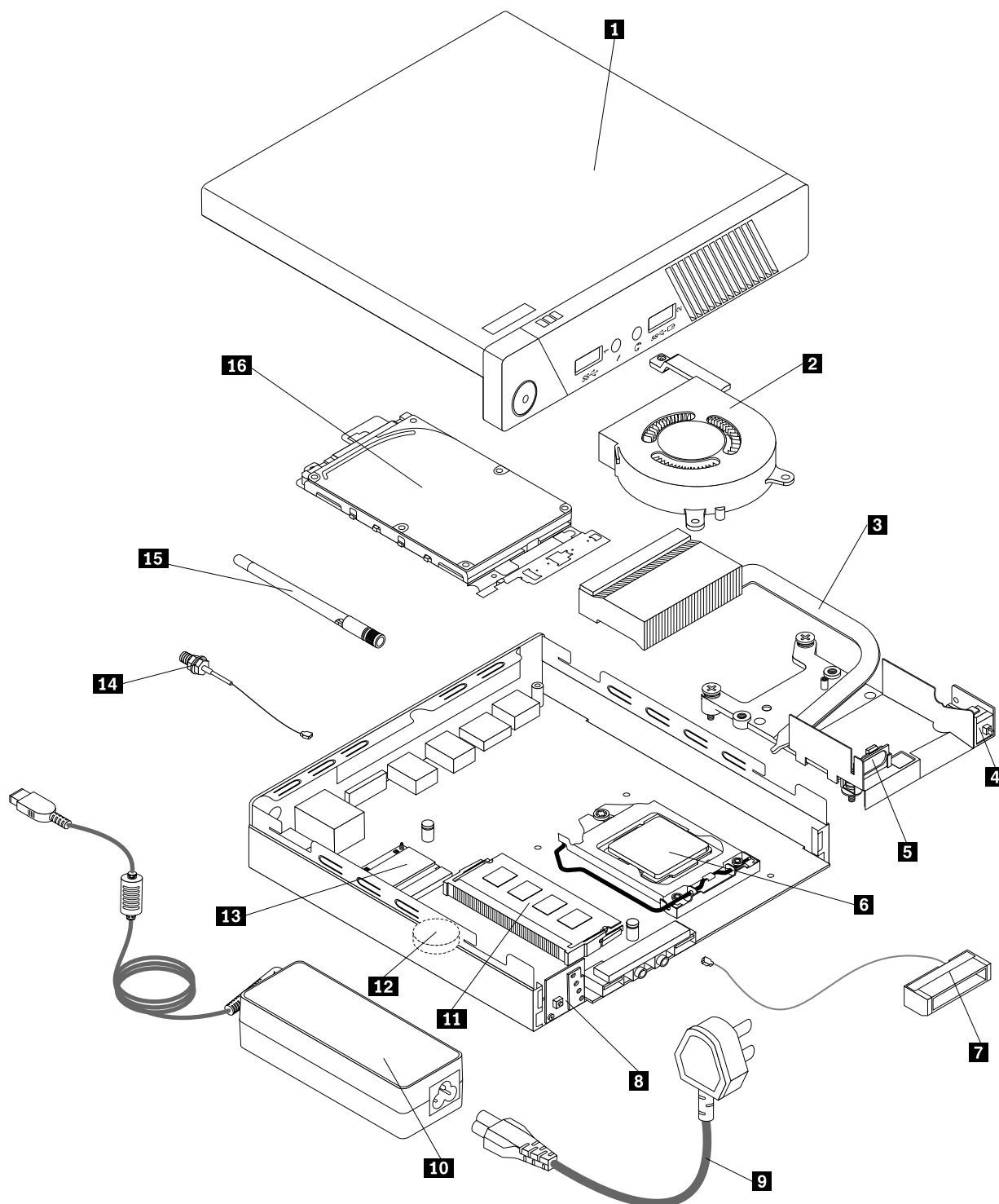
Abbildung 3. Positionen der Komponenten
