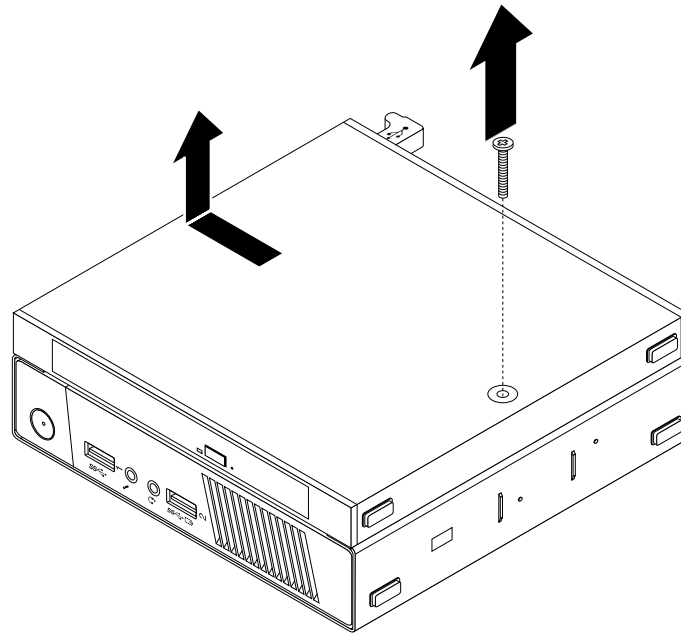
Abbildung 17. Gehäuse für das optische Laufwerk entfernen
