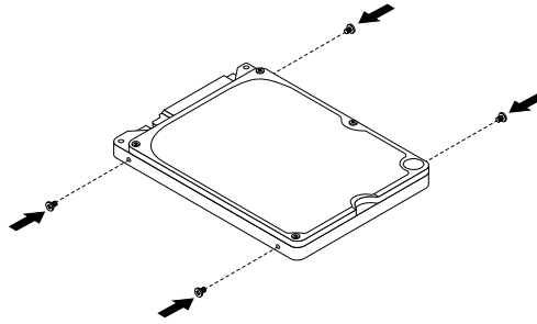
Abbildung 29. Vier Schrauben am Festplattenlaufwerk anbringen
