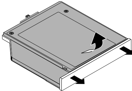
Abbildung 27. Adapter für das Festplattenlaufwerk aus der Adapterhalterung entfernen
