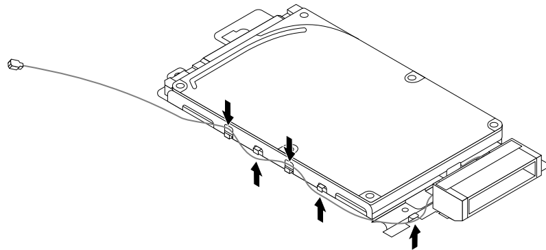
Abbildung 55. Kabel der vorderen Wi-Fi-Antenne verlegen
