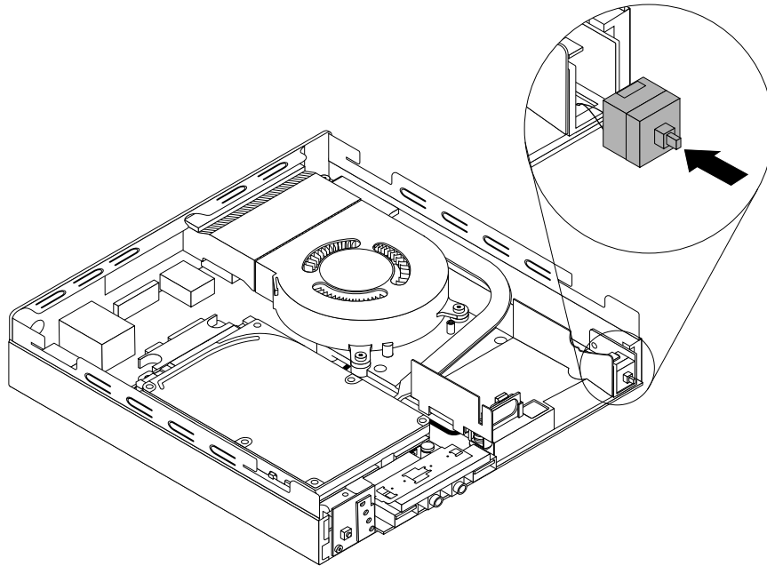
Abbildung 65. Schalter zur Abdeckungserkennung anbringen
