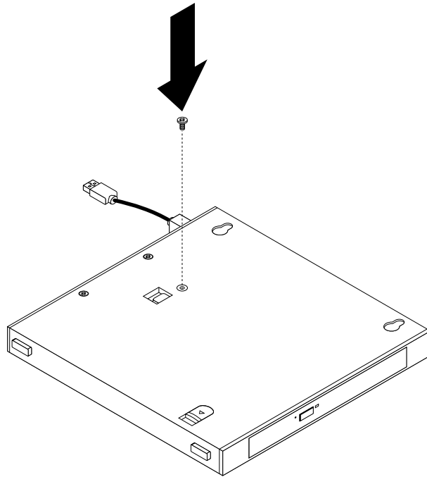
Abbildung 22. Schraube anbringen, mit der das optische Laufwerk gesichert ist
