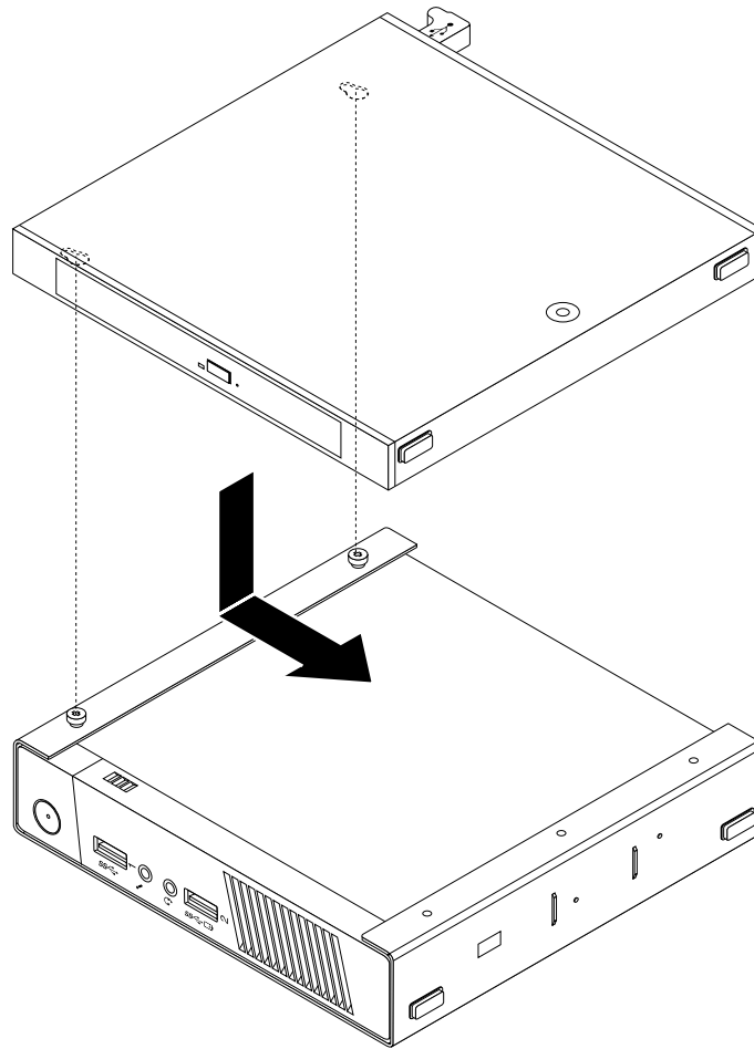
Abbildung 23. Gehäuse für das optische Laufwerk installieren
