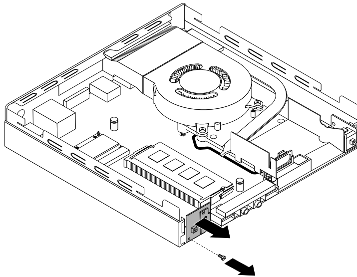
Abbildung 47. Netzschalter-Platine entfernen
