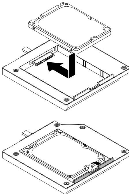
Abbildung 30. Ein neues Festplattenlaufwerk im Adapter installieren
