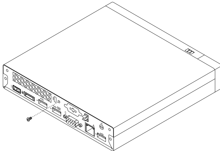
Abbildung 75. Schraube der Computerabdeckung anbringen
