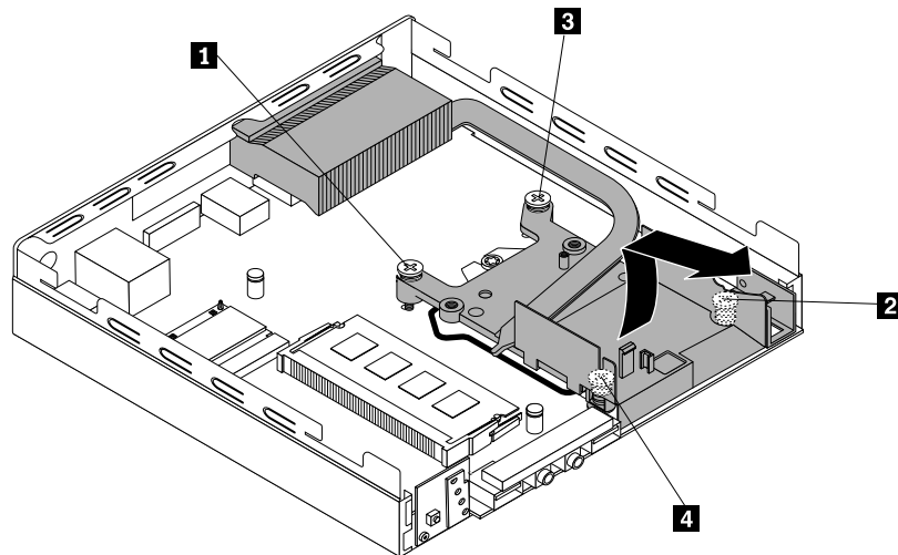
Abbildung 68. Temperaturmodul entfernen
