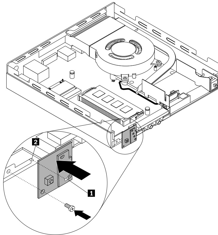
Abbildung 48. Netzschalter-Platine installieren
