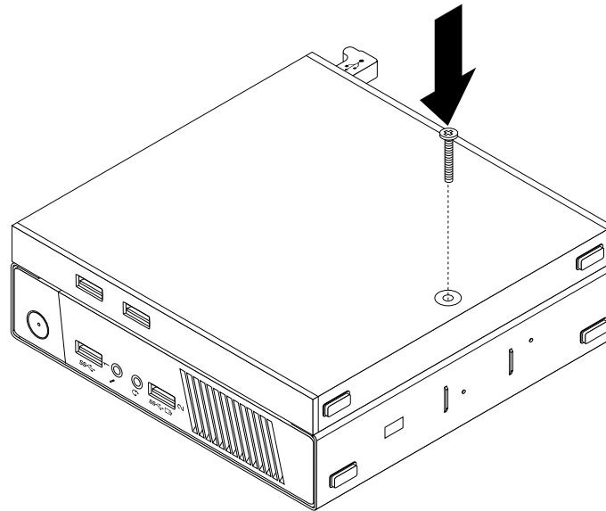
Abbildung 37. Schraube anbringen, um die E/A-Box zu sichern
