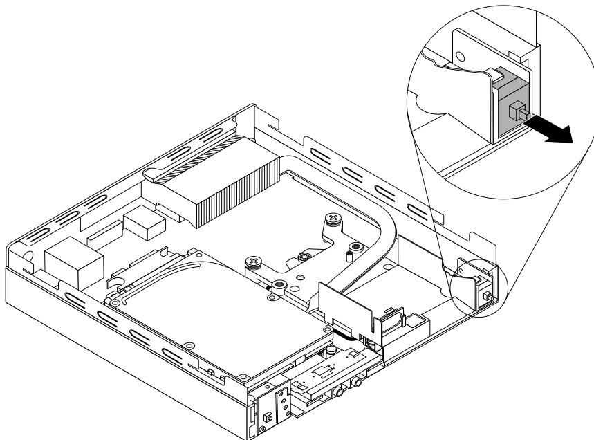
Abbildung 64. Schalter zur Abdeckungserkennung entfernen
