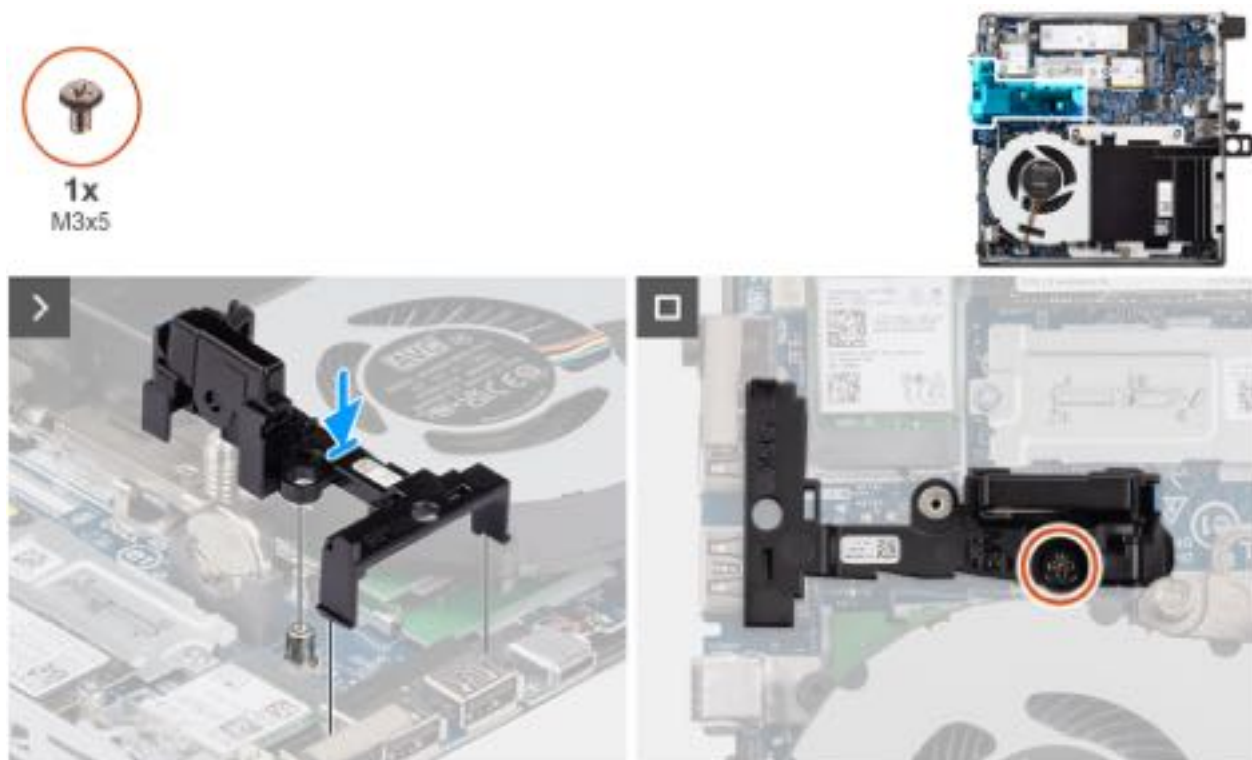
Abbildung 73. Installieren der Lautsprecherhalterung
