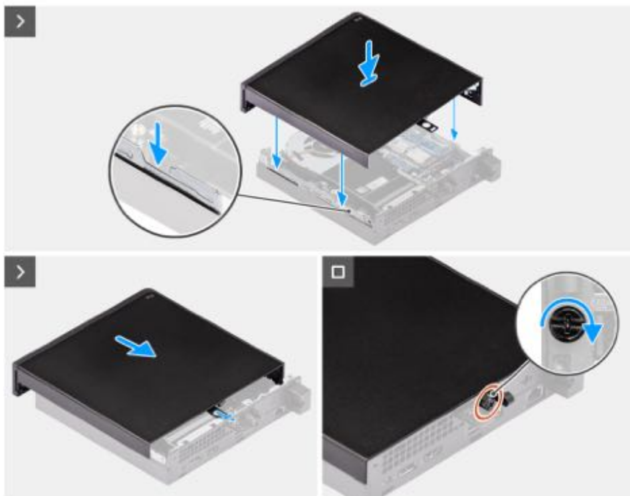
Abbildung 11. Anbringen der Seitenabdeckung
