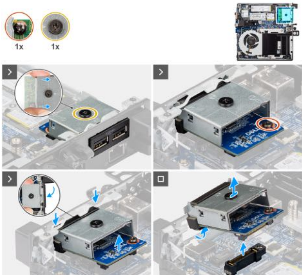
Abbildung 38. Entfernen des dualen USB-3.2-Gen2-Anschlussmoduls
