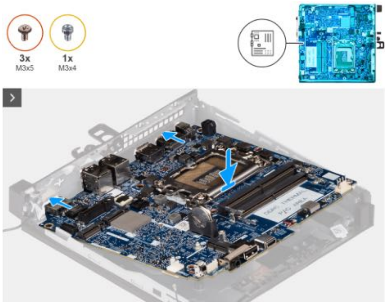
Abbildung 78. Einbauen der Systemplatine
