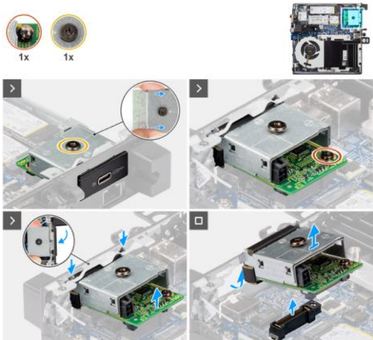
Abbildung 41. Entfernen des USB-Typ-C-Anschlussmoduls
