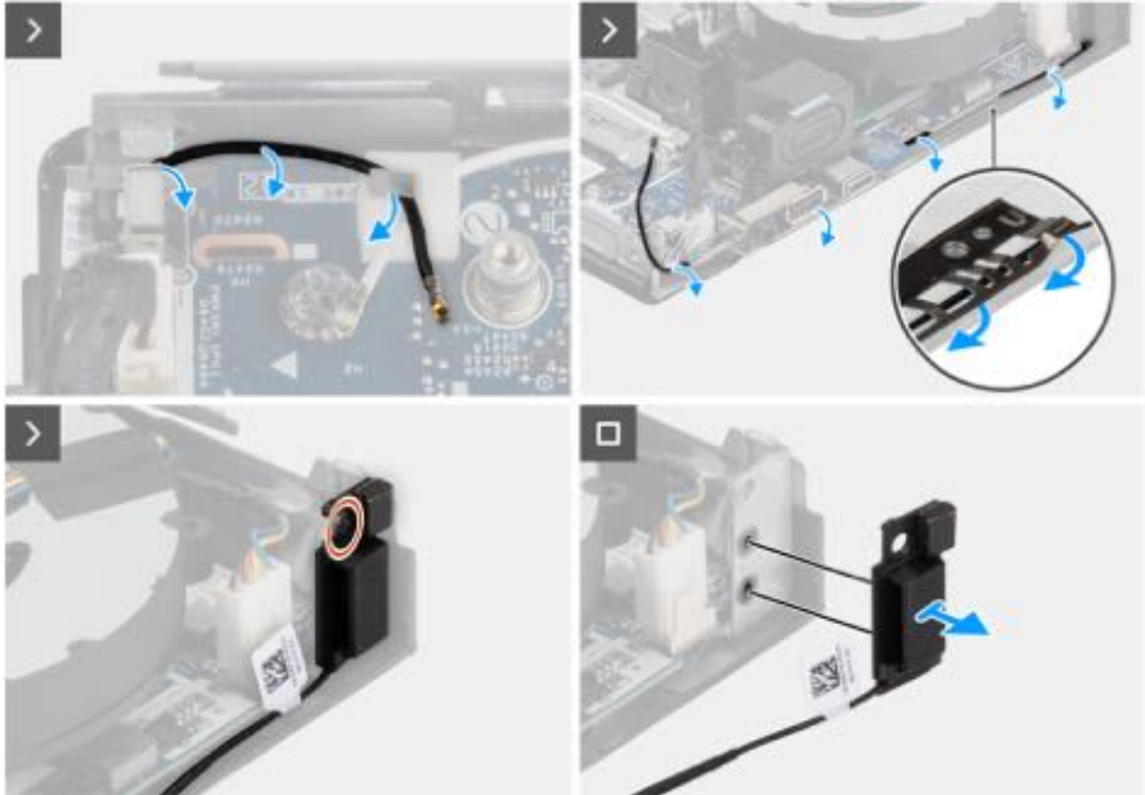
Abbildung 64. Entfernen des Antennenmoduls (schwarzes Kabel)
