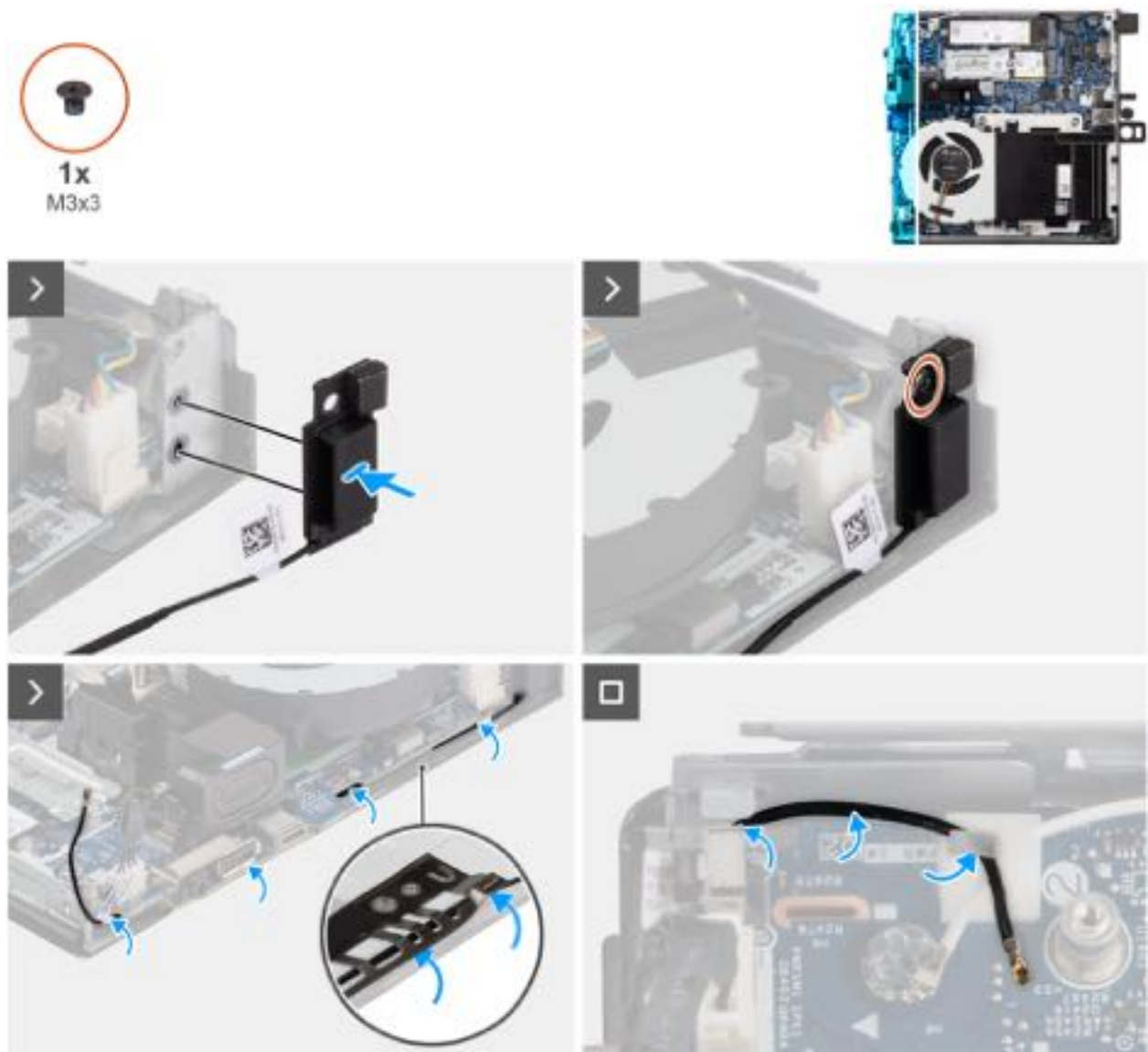
Abbildung 65. Einbauen des Antennenmoduls (schwarzes Kabel)
