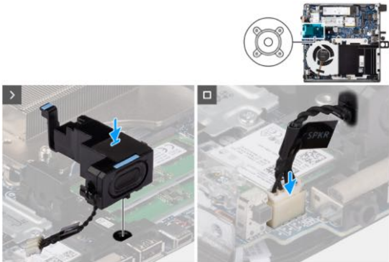
Abbildung 15. Einbauen des Lautsprechers
