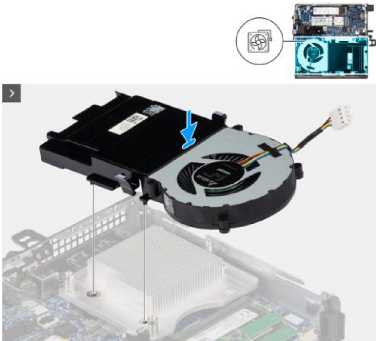
Abbildung 30. Einbauen des Lüfters
