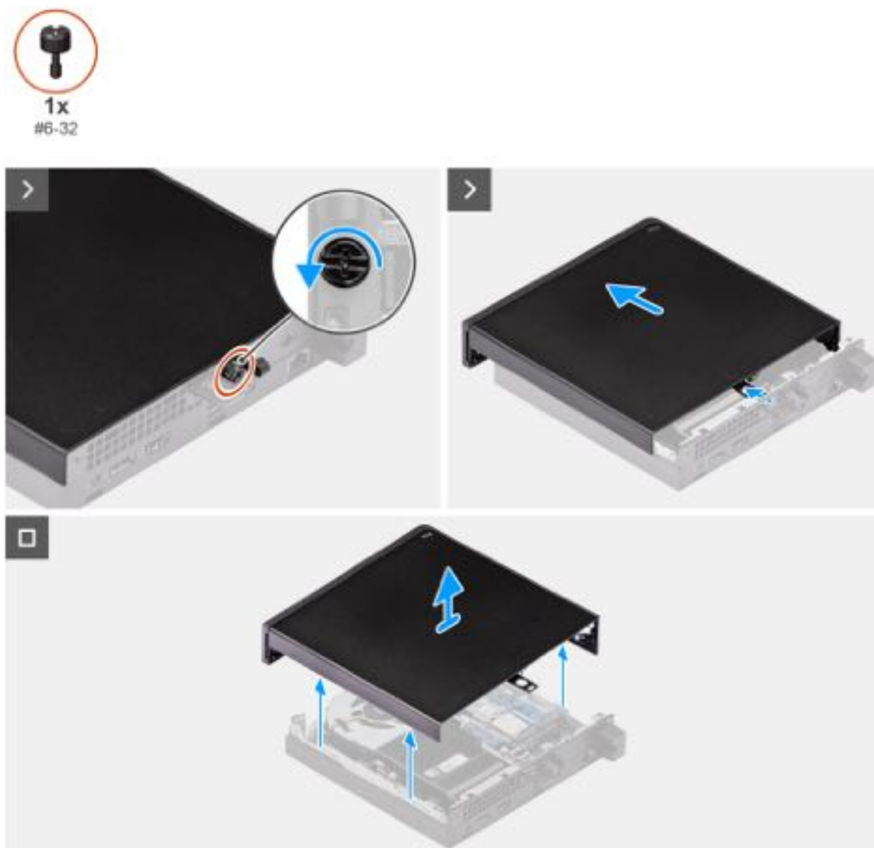
Abbildung 10. Entfernen der Seitenabdeckung
